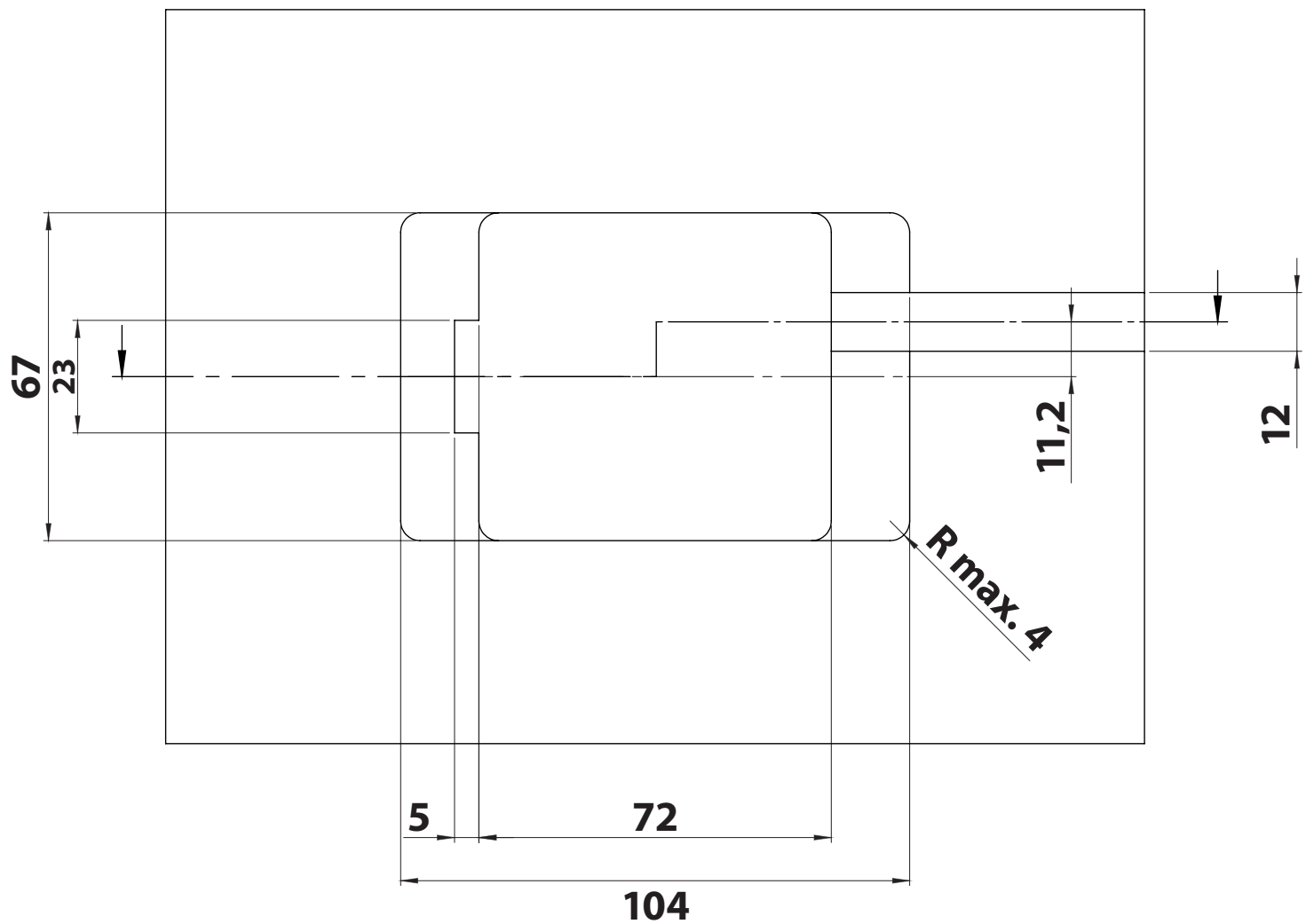
Unterseite der Tischplatte mit Maßen des Ausschnitts Bottom side of the table top with dimensions of the cut out
