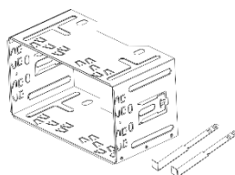
MONTERINGSSLOMME NØGLE TIL MONTERINGSFRIGIVELSE
